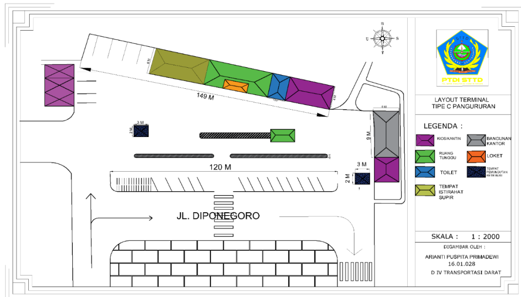
Gambar 3 Layout Terminal Setelah Penyesuaian
