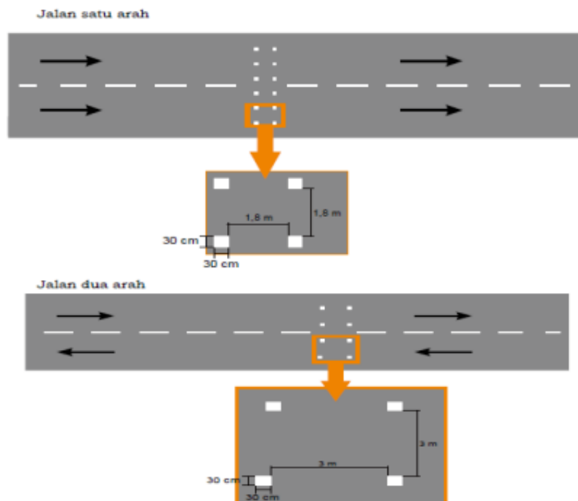
Gambar V. 16 Marka Penyebrang Untuk Pesepeda
