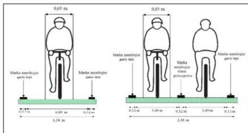
Gambar V. 13 Marka Jalur Sepeda
