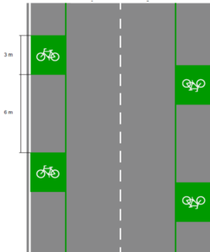
Gambar V. 13 Marka Jalur Sepeda
