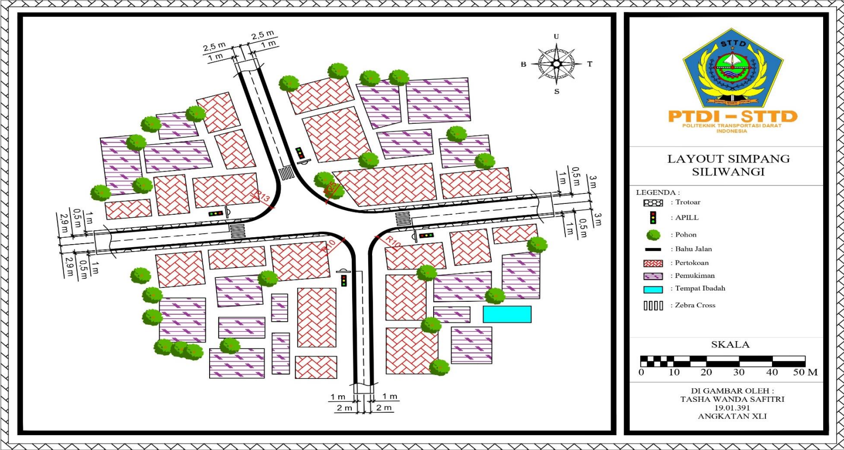
Lampiran 2 Layout Simpang Siliwangi
