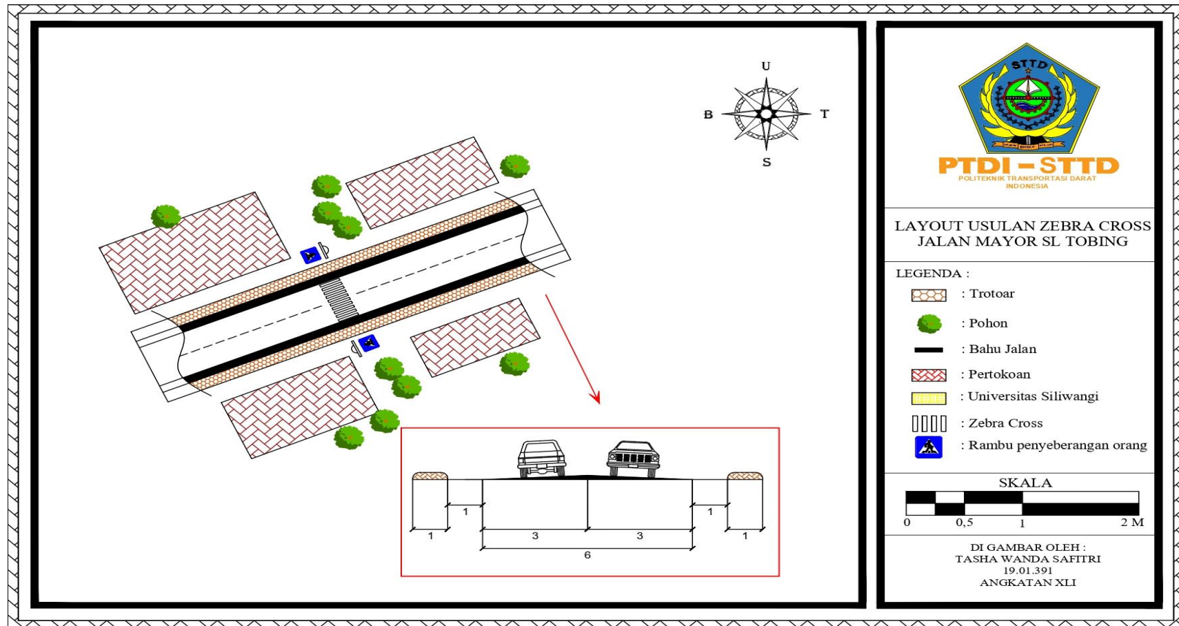
Lampiran 4 Layout Rekomendasi Fasilitas Penyeberangan Jalan Mayor SL Tobing
