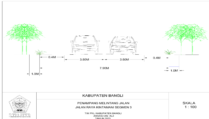
Gambar 2. 2 Penampang Melintang Jalan Raya Kintamani
