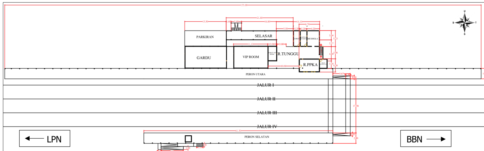
Gambar II. 5 Layout denah Stasiun Maguwo
