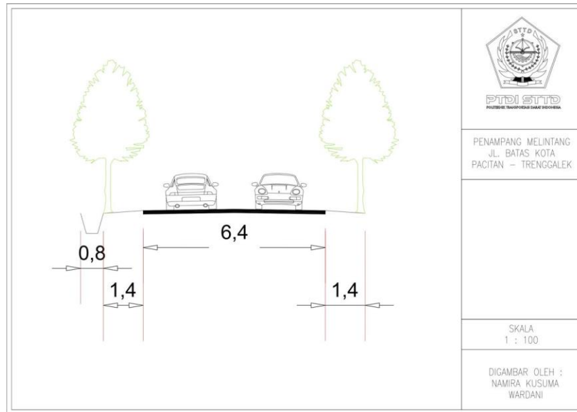
Gambar II. 8 Penampang Melintang Jalan Pacitan-Trenggalek 5
