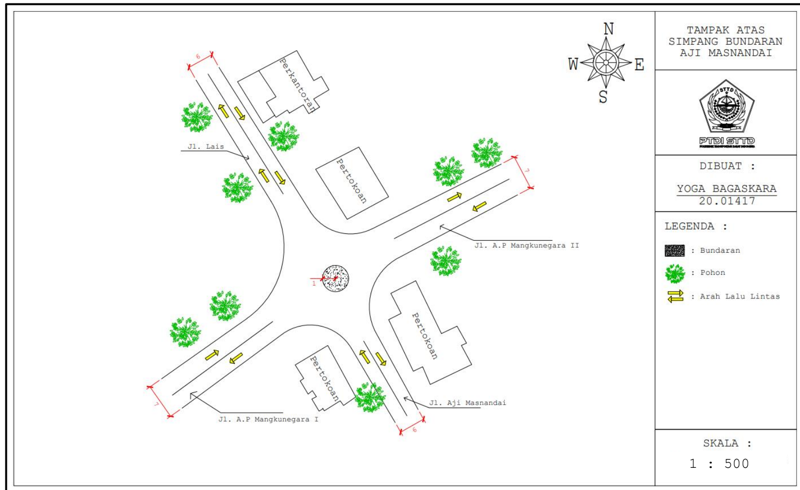
Gambar II. 6 Tampak Atas Simpang Bundaran Aji Masnandai
