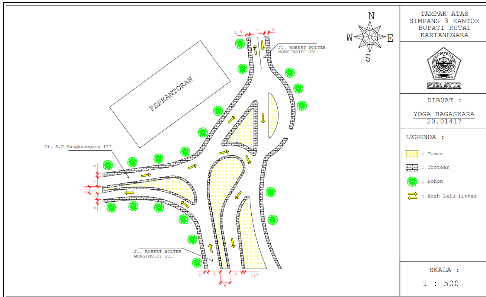
Gambar II. 4 Tampak Atas Simpang 3 Kantor Bupati Kutai Kartanegara
