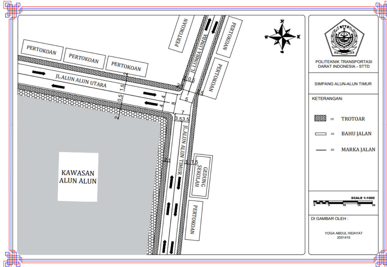
Gambar II. 4 Layout Simpang Alun-alun Timur
