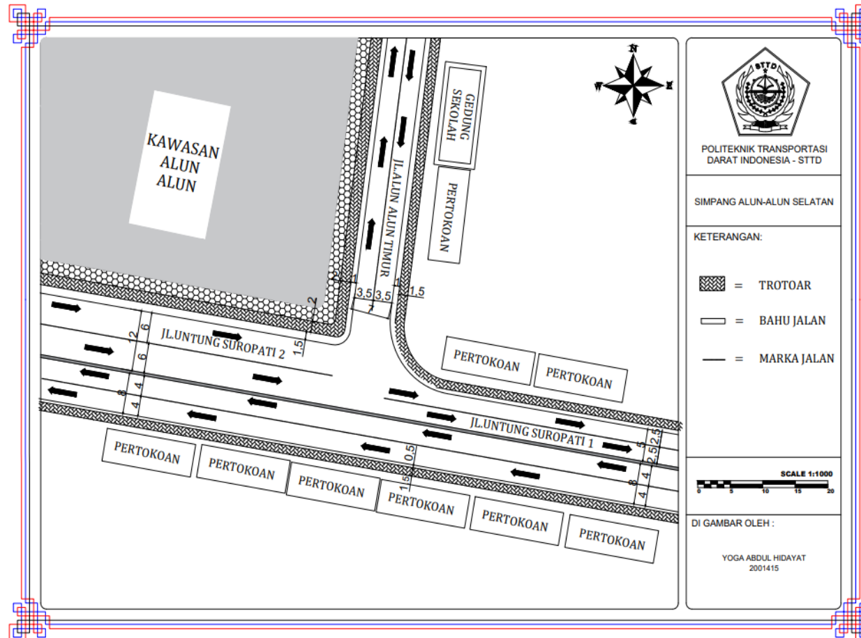
Gambar II. 5 Layout Simpang Alun-alun Selatan
